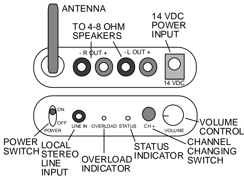
Fig. 1 WRA-50 AMPLIFIER
