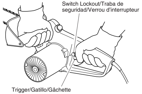
Figure 9 - Switch Lockout and Trigger Location Figura 9 - Ubicación del Bloqueo del Interruptor y el Gatillo Figure 9 - Emplacements du bouton du verrouillage d'interdiction de la gâchette et de la gâchette
