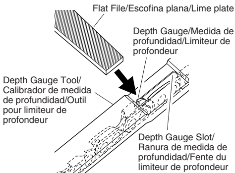
Figure 21 - Depth Gauge Tool On Chain Figura 21 - Calibrador de medida de profundidad en la cadena
