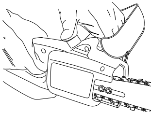
Figure 8 - Pressing Squeeze Bulb on Oil Cap to Oil Chain Figura 8 - Presione la Ampolla de Apriete en la Tapa del Aceite para Aceitar la Cadena Figure 8 - Comment presser la poire de graissage du bouchon de remplissage du carter d'huile pour huiler la chaîne
