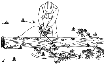
Figure 13 - Bucking Log With Entire Length On Ground Figura 13 - Trozado del tronco completamente apoyado en el suelo Figure 13 - Tronçonnage d'une bille qui repose entièrement au sol
