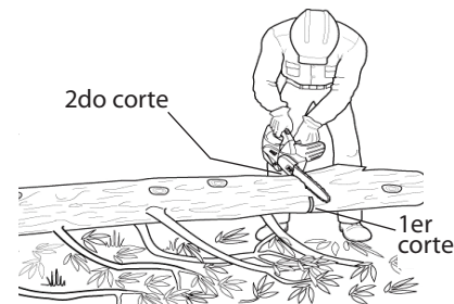
Figura 18 - Trozado del tronco apoyado sobre un solo extremo
