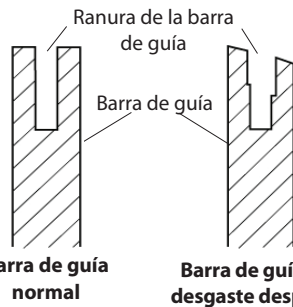
Figura 30 - Sección transversal de la barra de guía que ilustra el desgaste desparejo de la misma
