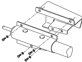
Figure 6 - Assembly of Pole Saw Brackets Figura 6 - Ensamble de Soportes de la Sierra de Pértiga Figure 6 - Assemblage des consoles de support de la scie à perche
