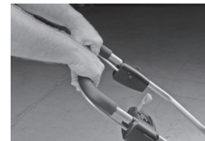
Figure 23 - Relevez la poignée de sécurité
