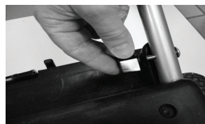
Figure 2 - Insérez les boulons connecteurs
