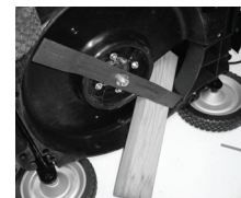
Figur6 25 - Acuña de la madera
