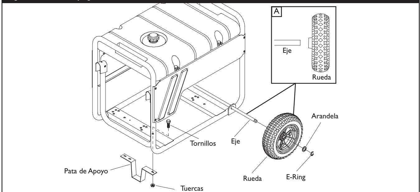
Figura 15 — Instale el Juego de Ruedas
