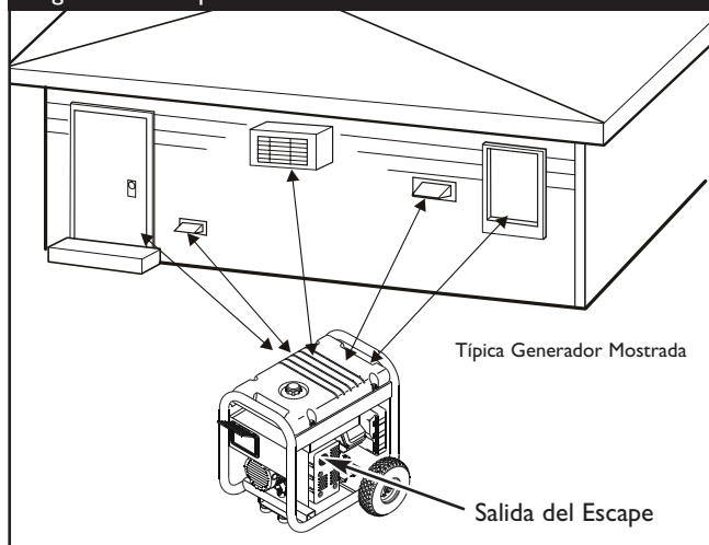
Figura 17 — Espacio Libre Alrededor del Generador
