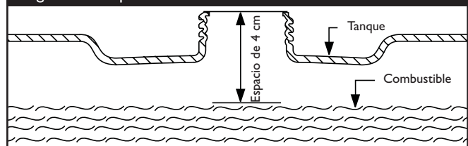
Figura 16 - Espacio de Combustible
