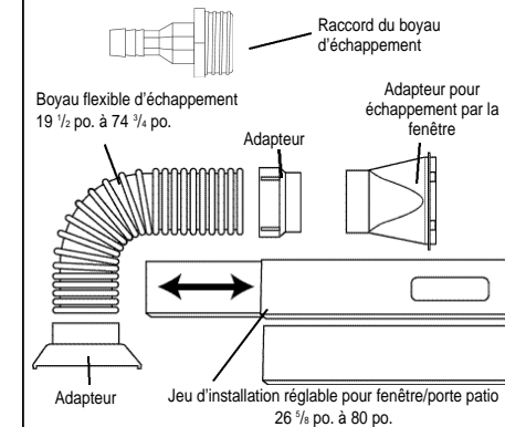
Fig. 1 Accessoires d'installation
