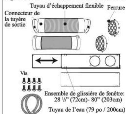
Fig. 1 ACCESSOIRES D'INSTALLATION
