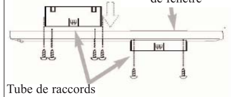
Fig. 2 L'arrière du panneau de fenêtre
