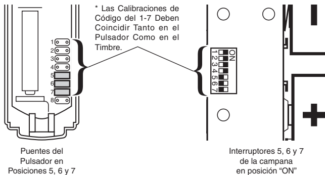
Figura 9 - Dentro del pulsador y de la campana
