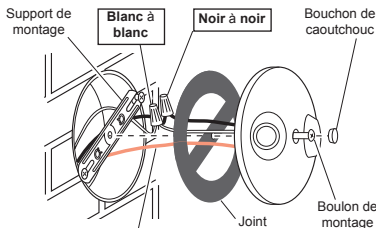
Câblage du projecteur
