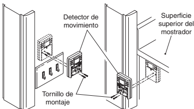
Fijación del detector de movimiento directamente a la pared
