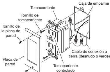
Instalación del receptor con tomacorriente
