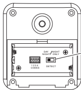
Detector de movimiento para uso exterior (Vista posterior)
